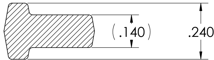
SECTION A-A SCALE 4 : 1
