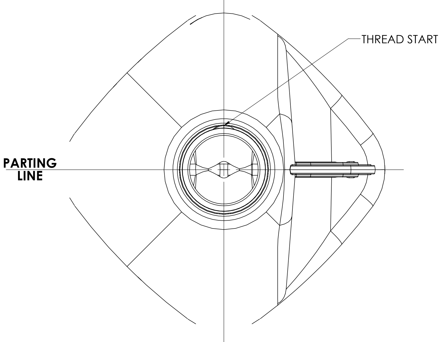
SECTION A-A SCALE 4 : 1
